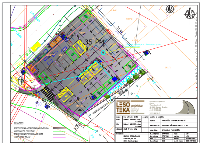
Situacija ureditve parkirišča in javne tržnice
