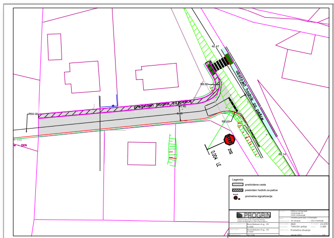
Prometna ureditev ulice Cerkvjenjak-Govedič
